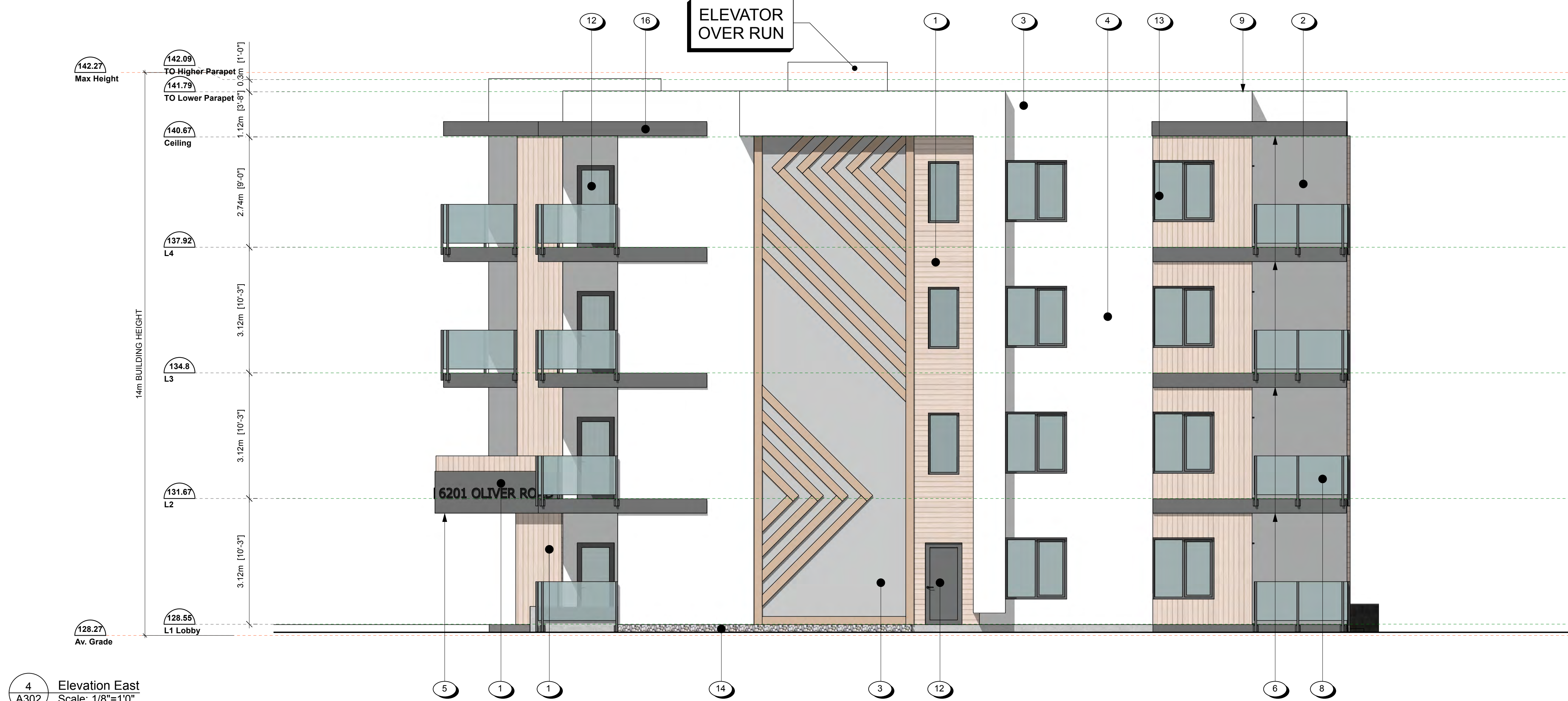
3 Elevation North A302 Scale: 1/8"=1'-0"
